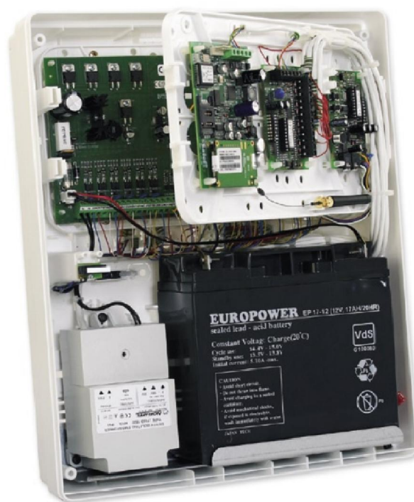
Príklad umiestnenia zariadení do skrinky OPU-3 P
